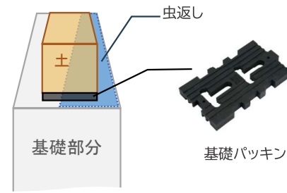
(図1:虫返しの上に基礎パッキンイメージ)
