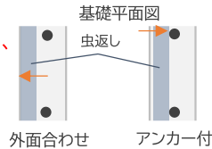
(図3:基礎外面合わせ)
