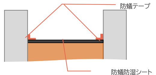
(図4: 防蟻テープ施工位置)
