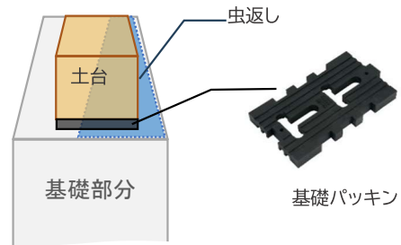
(図1: 虫返しの上に基礎パッキンイメージ)
